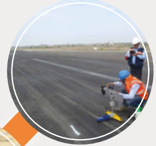
PÉNDULO TRRL
